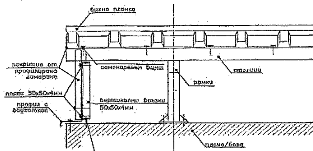
стална ферма с профили 50x50x4mm и покритие от профилна ламарина за затваряне на отвор
