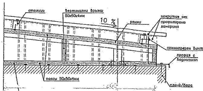
стална ферма с профили 50x50x4mm и покритие от профилна ламарина за затваряне на отвор
