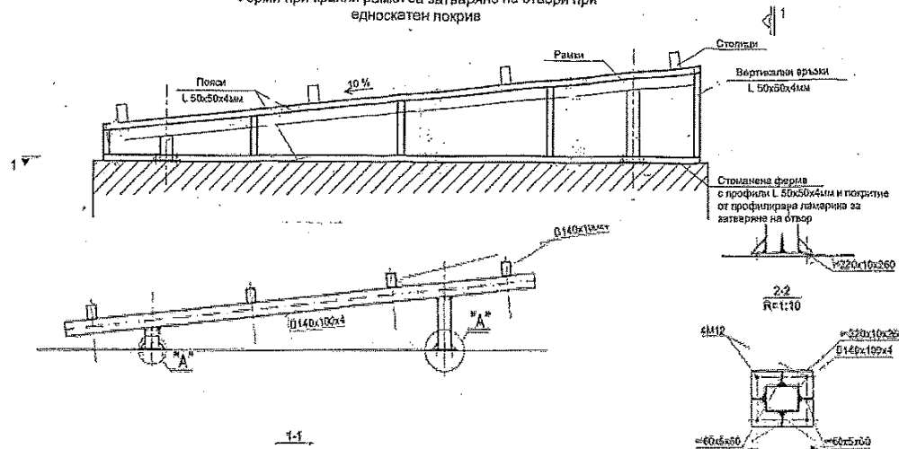
Ферми при крайни рамки за затваряне на отвори при едноскатен покрив
